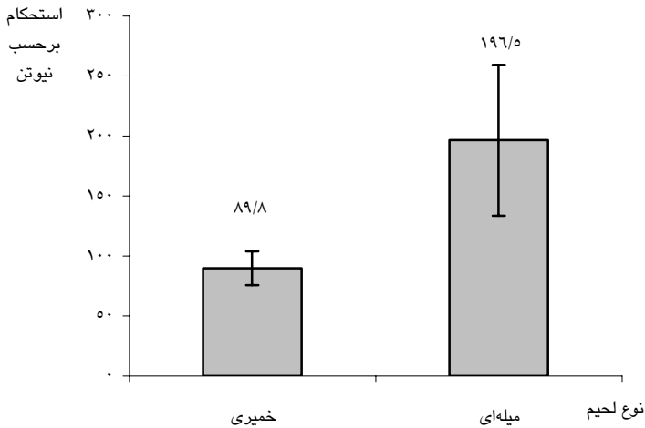
نمودار ۲: مقایسه میانگین استحکام خمشی لحیم خمیری با میله‌ای
